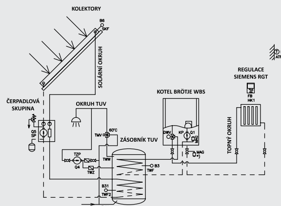
SCHÉMA PRO ZAPOJENÍ SOLÁRNÍCH SETŮ S KOTLEM BRÖTJE WBS-F
