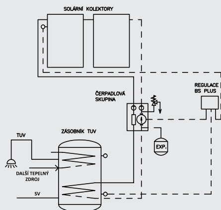
SCHÉMA PRO ZAPOJENÍ SAMOSTATNÝCH SOLÁRNÍCH SETŮ
