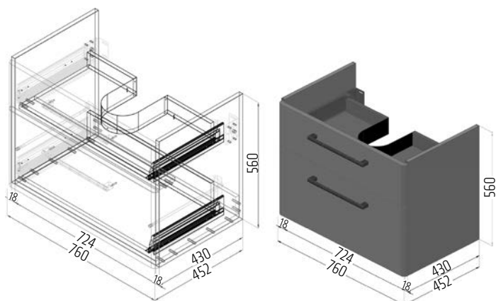
Skříňka se 2 zásuvkami k umyvadlu 80 cm
