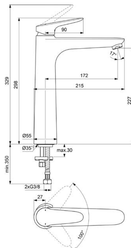
Umyvadlová stojánková bez výpustí, XL
