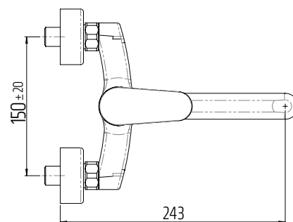
Umyvadlová nástěnná s otočným ramínkem 180 mm
