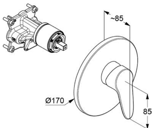
Sprchová podomítková bez podomítkového tělesa
