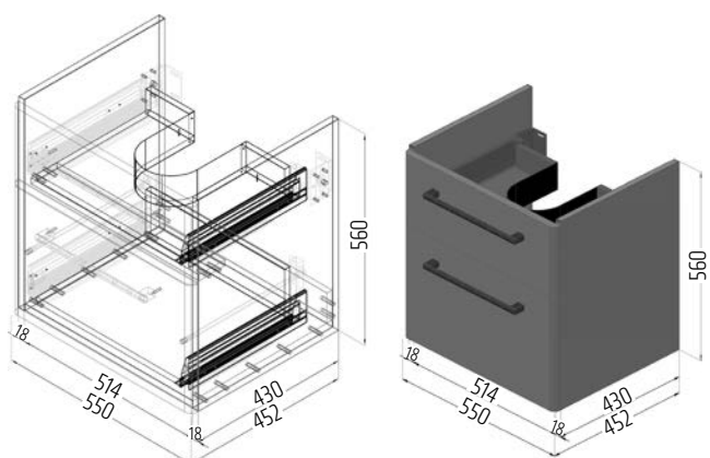
Skříňka se 2 zásuvkami k umyvadlu 60 cm
