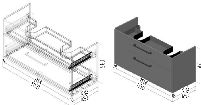
Skříňka pod dvojumyvadlo 120 cm dělená vnitřní plocha dva šuplíky
