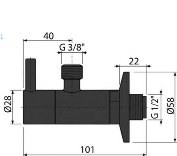
Ventil rohový 1/2"x3/8" kulatý
