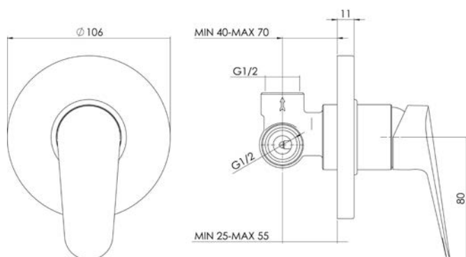
Sprchová podomítková včetně podomítkového tělesa
