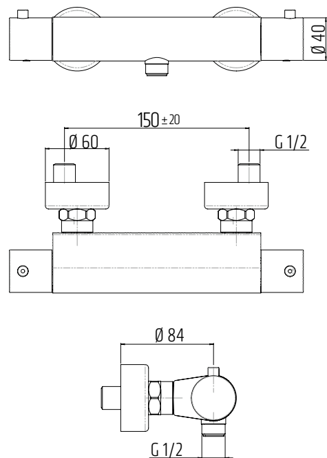
Termostatická sprchová nástěnná
