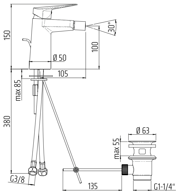
Bidetová s výpustí
