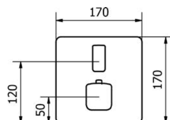
Termostatická podomítková vrchní díl s přepínáním
