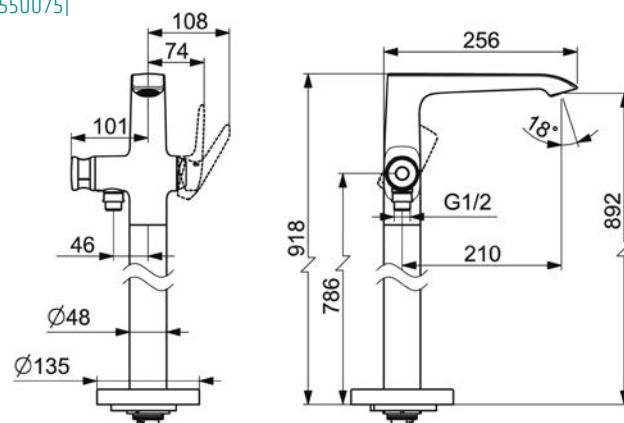
Vanová volně stojící
