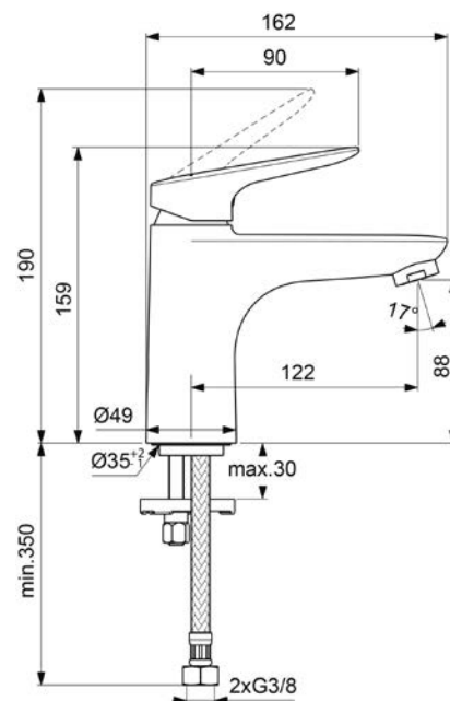
Umyvadlová bez výpustí
