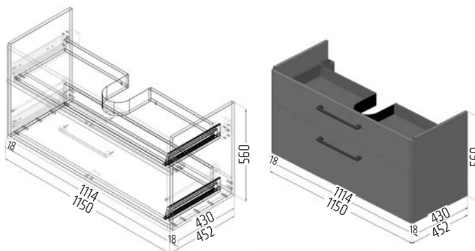
Skříňka pod dvojumyvadlo 120 cm nedělená vnitřní plocha dva šuplíky
